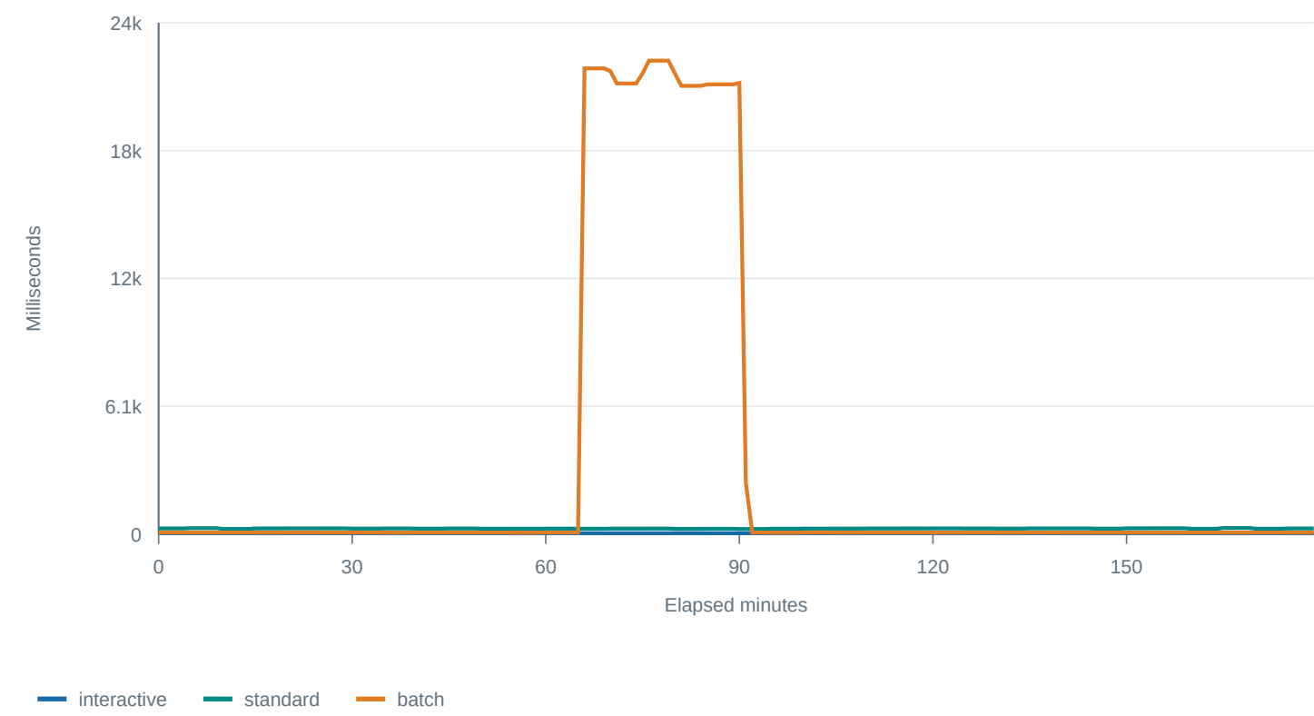
Tenant TTFT P95
