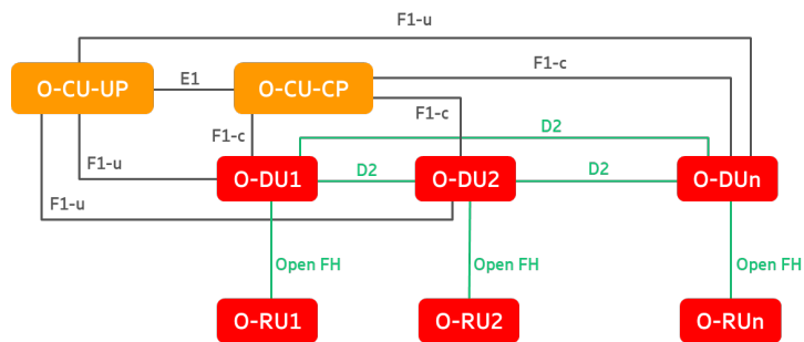
A.6-1: Inter O-DU CA
