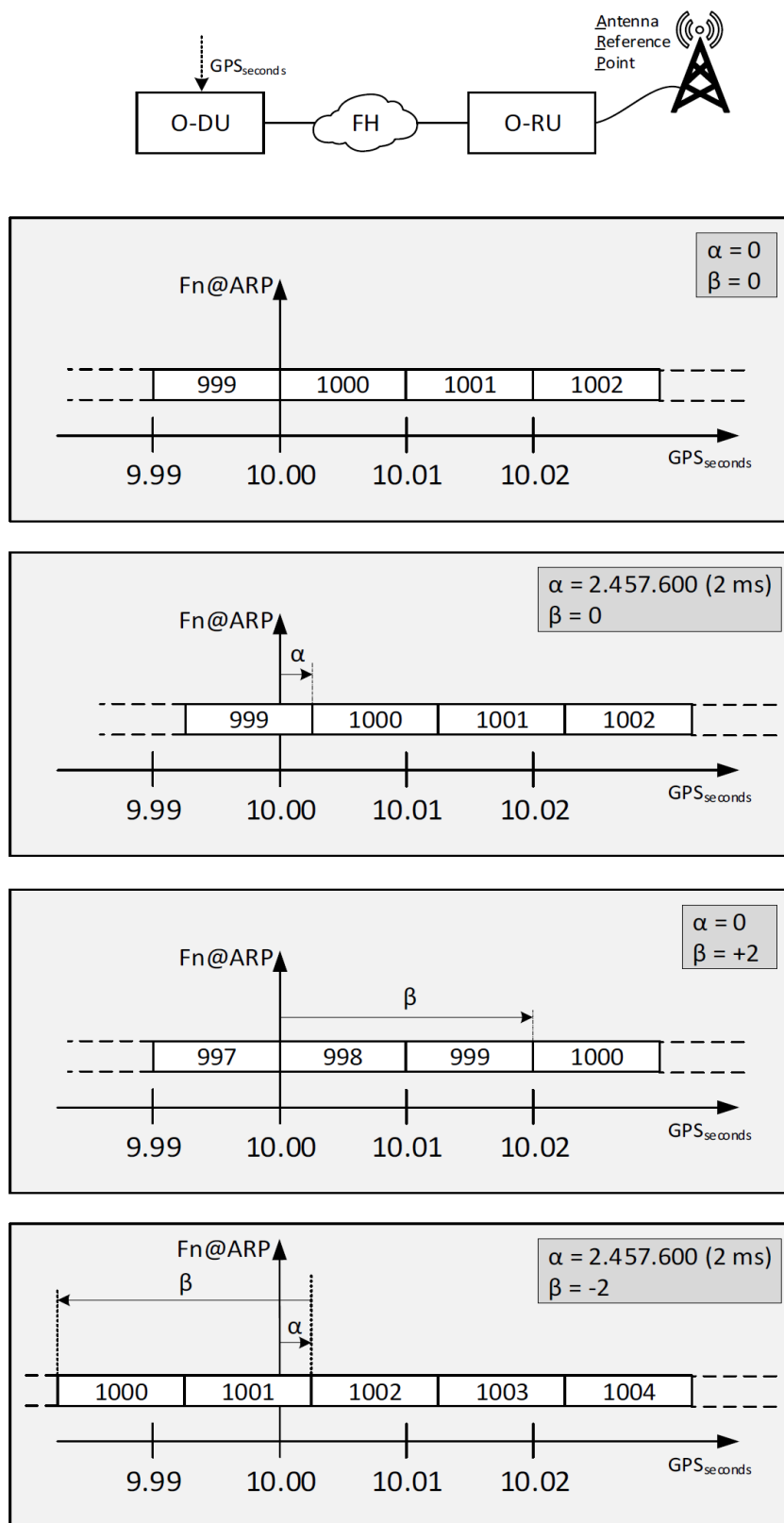
Figure 11.7.2-1: \alpha and \beta parameter example
