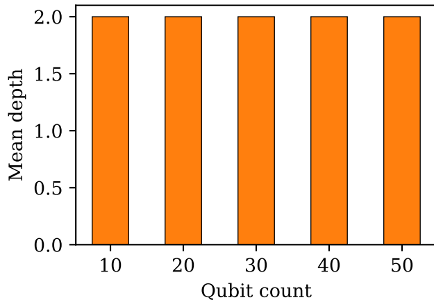
Pytket
