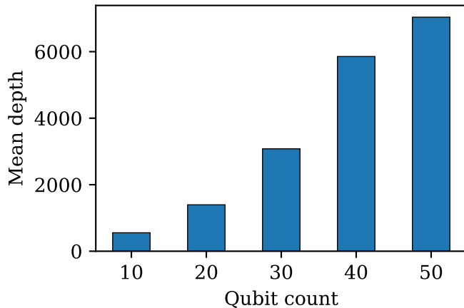
Qiskit
