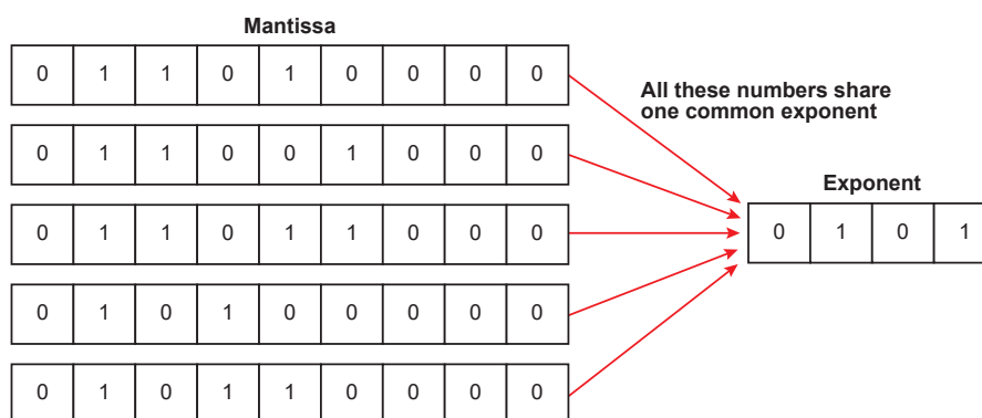
Σχήμα 0-4 Η αναπαράσταση κινητής υποδιαστολής ομάδας δεδομένων.
