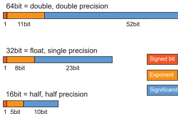
Σχήμα 0-3 Αναπαράσταση κινητής υποδιαστολής μισής, απλής και διπλής ακριβείας σύμφωνα με το πρότυπο IEEE 754.
