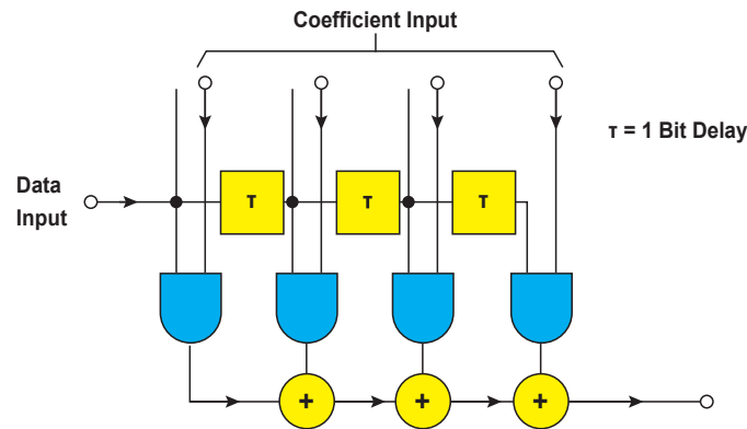
Σχήμα 0-8 Σχηματικό διάγραμμα σειριακού πολλαπλασιαστή (Freeny, Σχήμα 11).
