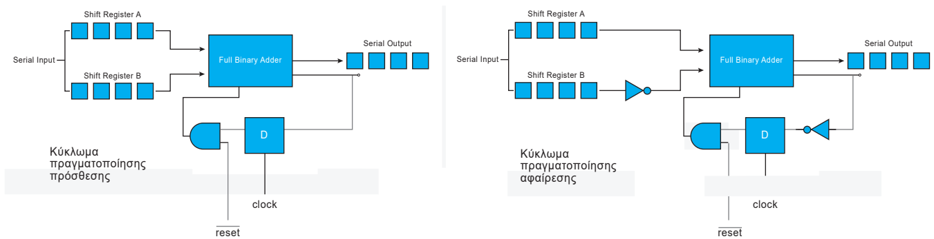
Σχήμα 0-3 Το δομικό διάγραμμα του σειριακού αθροιστή (αριστερή εικόνα) και οι τροποποιήσεις που πρέπει να γίνουν έτσι ώστε αντί για πρόσθεση να εκτελεί αφαίρεση (δεξιά εικόνα).
