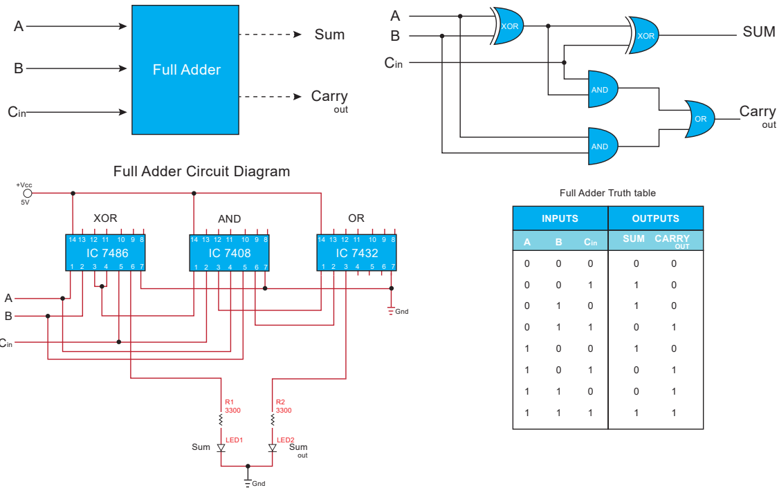
Σχήμα 0-2 Το δομικό διάγραμμα του πλήρους αθροιστή μαζί με το λογικό διάγραμμα και το αντίστοιχο λογικό κύκλωμα.
