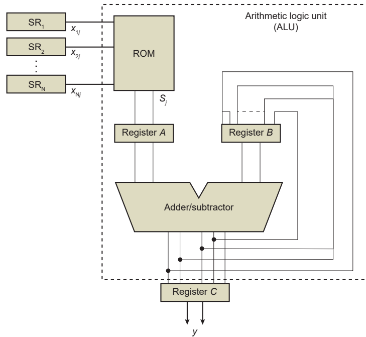
Σχήμα 0-10 Κύκλωμα καταμεμημένου υπολογισμού αθροίσματος γινομένων.
