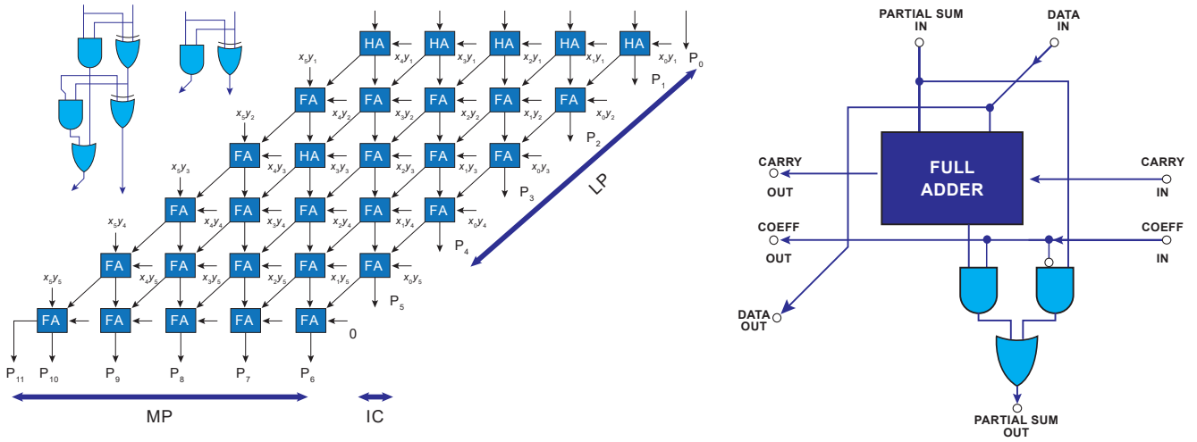
Σχήμα 0-9 Σχηματικό διάγραμμα παράλληλου πολλαπλασιαστή (αριστερή εικόνα) και κελί Hoffmann (δεξιά εικόνα) (Freeny, Σχήμα 15).
