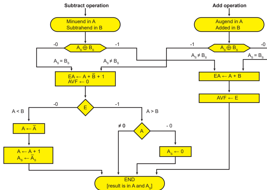
Σχήμα 0-1 Οι διαδικασίες πρόσθεσης και αφαίρεσης ακεραίων που είναι εκπεφρασμένοι στη μορφή πρόσημου μεγέθους (Chauhan P, Addition and Subtraction , https://www.naukri.com/code360/library/addition-and-subtraction ).
