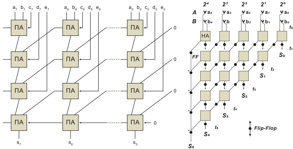
Σχήμα 0-4 Αθροιστής διατήρησης κρατούμενου (αριστερή εικόνα) και αθροιστής που λειτουργεί με διοχέτευση (δεξιά εικόνα).
