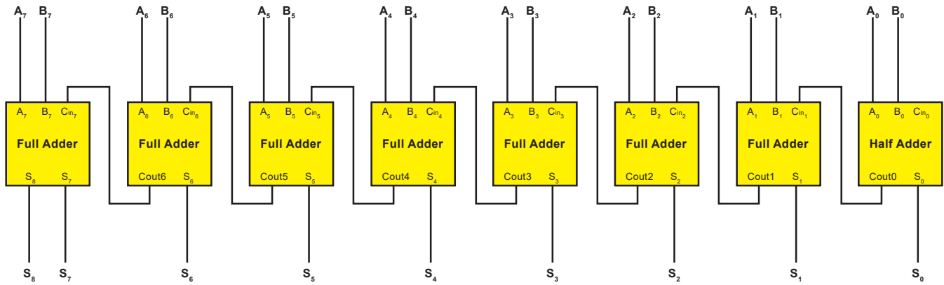
Σχήμα 0-6 Σχηματικό διάγραμμα παράλληλου αθροιστή που επιτρέπει την πρόσθεση δυαδικών αριθμών μήκους οκτώ bits.
