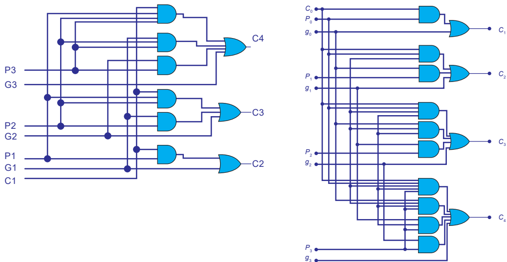
Σχήμα 0-5 Το συνδυαστικό κύκλωμα που επιτρέπει τον εκ των προτέρων υπολογισμό των κρατούμενων για την πρόσθεση αριθμών με μήκος N = 3 bits (αριστερή εικόνα) και N = 4 bits (δεξιά εικόνα). Οι εισόδους p_i και g_i που χρησιμοποιούνται σε αυτά τα κυκλώματα, ορίζονται ως p_i = x_i \cdot y_i [παραγωγή κρατούμενου (carry generate)] και g_i = x_i \otimes y_i ( i = 1, 2, \dots, N ) [διάδοση κρατούμενου (carry propagate)].
