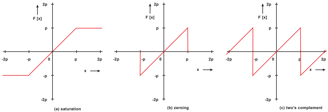
Σχήμα 0-1 Χαρακτηριστικές εισόδου - εξόδου για τους τρεις μηχανισμούς ανάκαμψης από υπερχείλιση που είναι ο κορεσμός (αριστερή εικόνα), ο μηδενισμός (μεσαία εικόνα) και η πρόσθεση συμπληρώματος ως προς 2 (δεξιά εικόνα).
