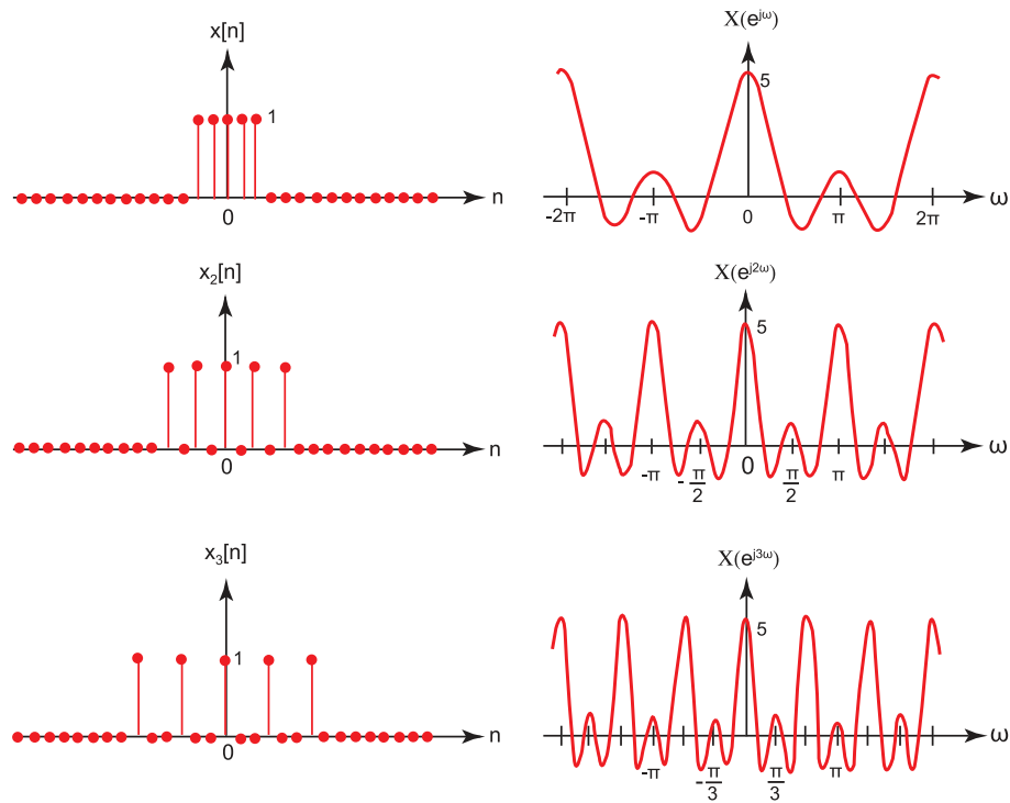
Σχήμα 0-1 Η μεταβολή του σήματος x_k[n] και του μετασχηματισμού του κατά Fourier \mathcal{X}_k(e^{j\omega}) για διαφορετικές τιμές της παραμέτρου k .
