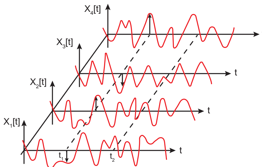
Σχήμα 0-1 Μία συλλογή συναρτήσεων, οι οποίες συνιστούν από κοινού μία τυχαία διεργασία (Razdolsky L, Random Processes, in Probability-Based Structural Fire Load , Cambridge University Press, 2014, pp. 89-136, Σχήμα 3.1).
