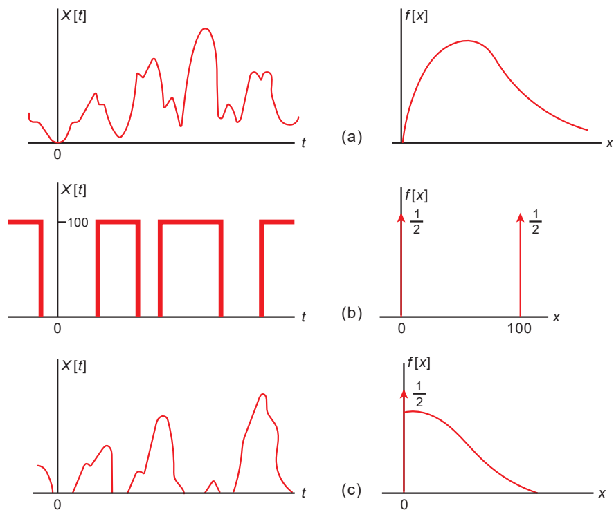
Σχήμα 0-2 Παράδειγμα συνεχούς [εικόνα (α)], διακριτής [εικόνα (β)] και μικτής [εικόνα (γ)] τυχαίας διεργασίας. Για κάθε τύπο διεργασίας, η αριστερή εικόνα απεικονίζει μία τυπική συνάρτηση - δείγμα της διεργασίας, ενώ η δεξιά εικόνα απεικονίζει την αντίστοιχη συνάρτηση πυκνότητας πιθανότητας.
