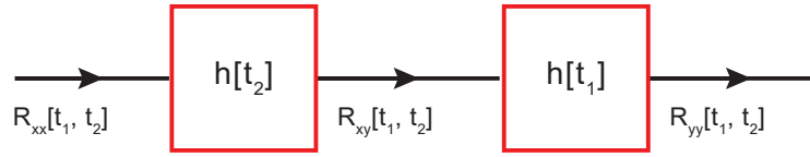
Σχήμα 0-2 Η συσχέτιση ανάμεσα στις συναρτήσεις R_{xx}(t_1, t_2) και R_{yy}(t_1, t_2) (Papoulis & Pillai, Σχήμα 9.8β).
