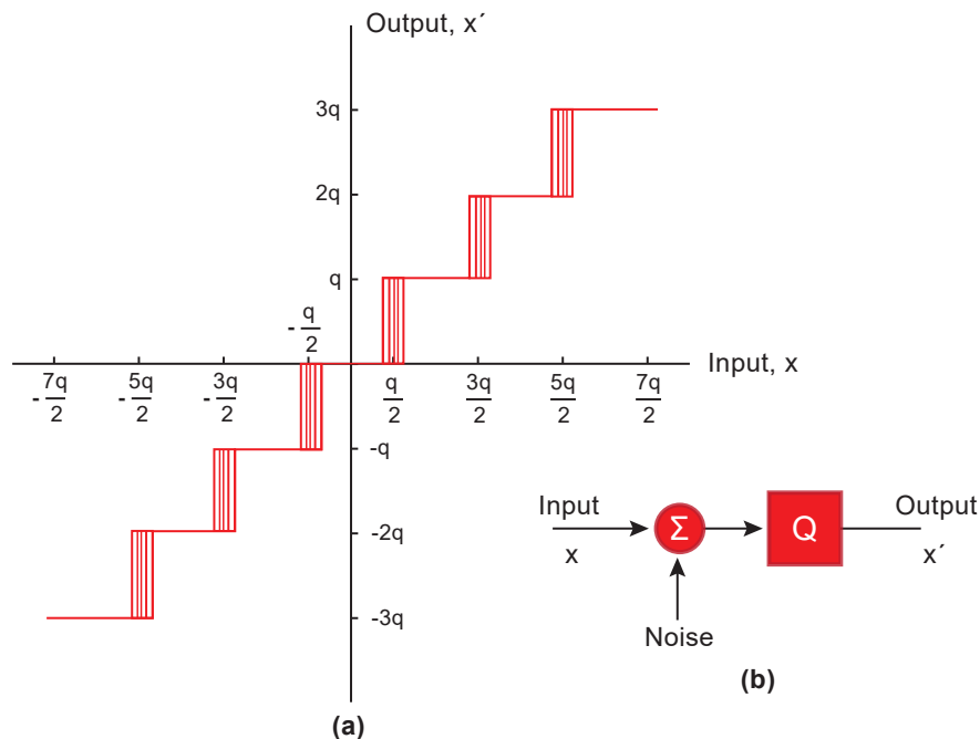
Σχήμα 0-3 Πραγματικός κβαντιστής που χαρακτηρίζεται από την ύπαρξη θορύβου (Widrow & Kollár, Σχήμα 1.7).
