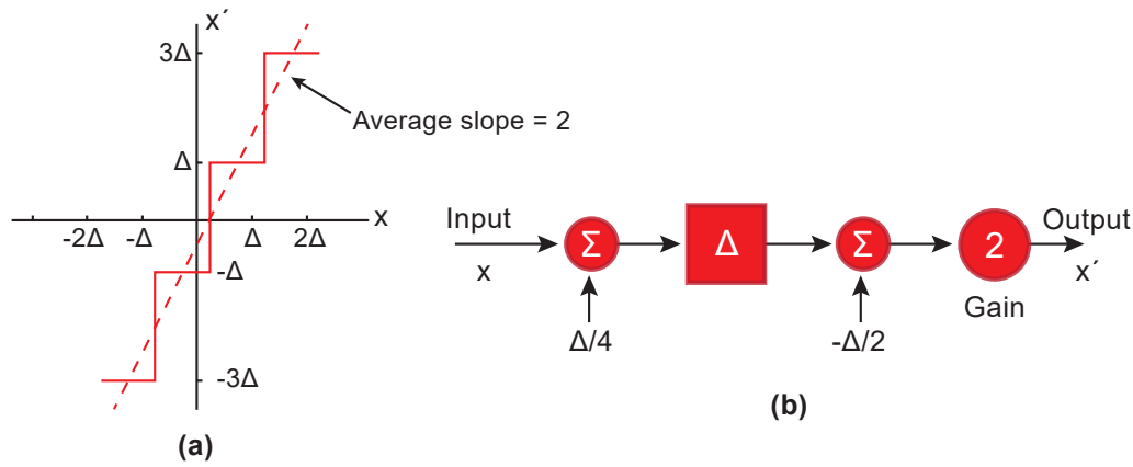
Σχήμα 0-2 Χαρακτηριστική καμπύλη κβαντιστή με διαφορετικά χαρακτηριστικά που προκύπτει συνδυάζοντας τον κβαντιστή με τα κατάλληλα στοιχεία (Widrow & Kollár, Σχήμα 1.3).
