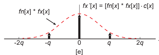
Σχήμα 0-6 Η διαδικασία της δειγματοληψίας επιφάνειας (Widrow & Kollár, Σχήμα 4.2).
