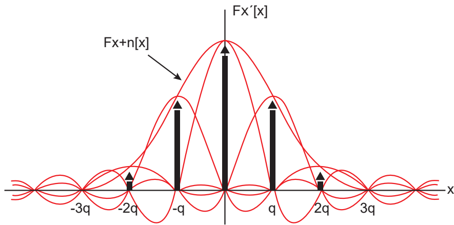
Σχήμα 0-7 Ανακατασκευή της πυκνότητας πιθανότητας f_x(x) της εισόδου x του κβαντιστή, από την πυκνότητα πιθανότητας f_y(y) της εξόδου του κβαντιστή y = Q(x) .
