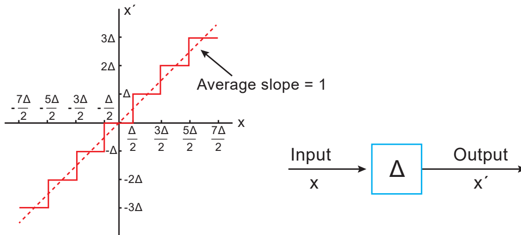
Σχήμα 0-1 Η τυπική χαρακτηριστική καμπύλη κβαντιστή με την περιοχή λειτουργίας να προσεγγίζεται από ευθεία y = x με κλίση ίση με τη μονάδα, στο όριο \Delta \rightarrow 0 .
