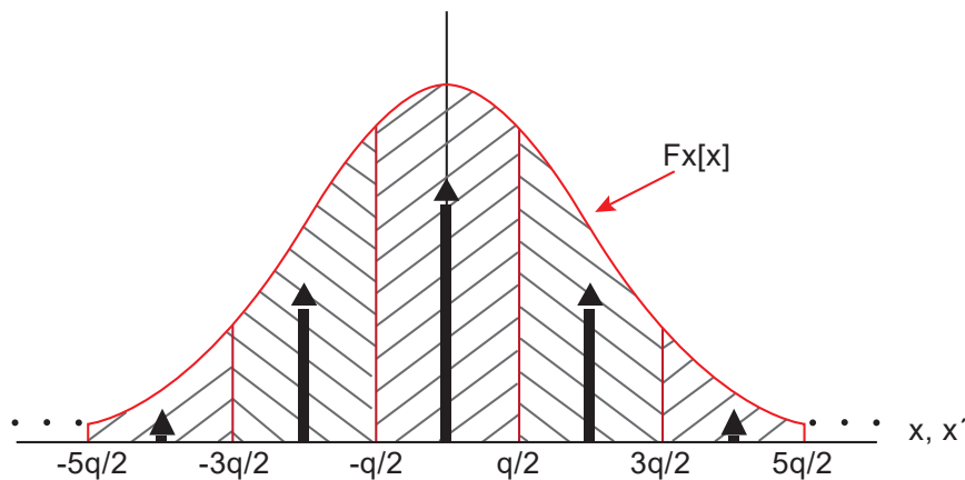
Σχήμα 0-5 Ο τρόπος κατασκευής της συνάρτησης πυκνότητας πιθανότητας f_y(y) (Widrow & Kollár, Σχήμα 4.1).
