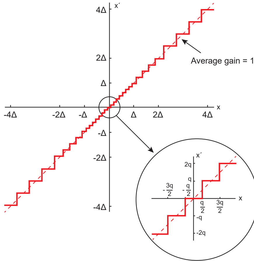
Σχήμα 0-1 Τυπική χαρακτηριστική εισόδου / εξόδου κβαντιστή κινητής υποδιαστολής (Widrow & Kollár, Σχήμα 12.3).
