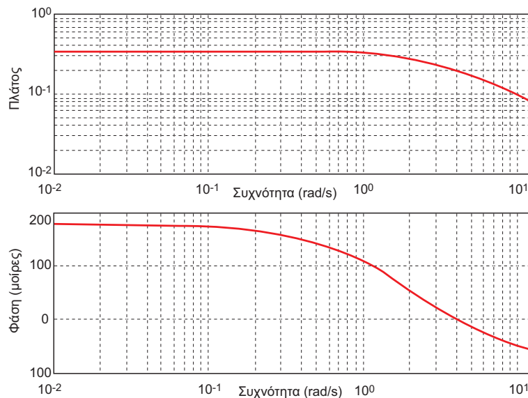
Σχήμα 0-1 Η απόκριση πλάτους και φάσης του συστήματος.
