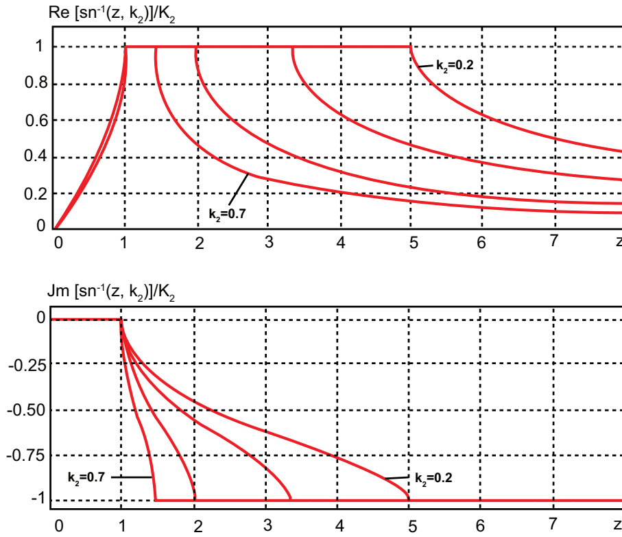
Σχήμα 0-3 Μεταβολή του πραγματικού και του φανταστικού μέρους της συνάρτησης \text{sn}^{-1}(z, k_2) για τιμές ελλειπτικού μέτρου k_2 = 0.2, 0.3, 0.5, 0.7 .
