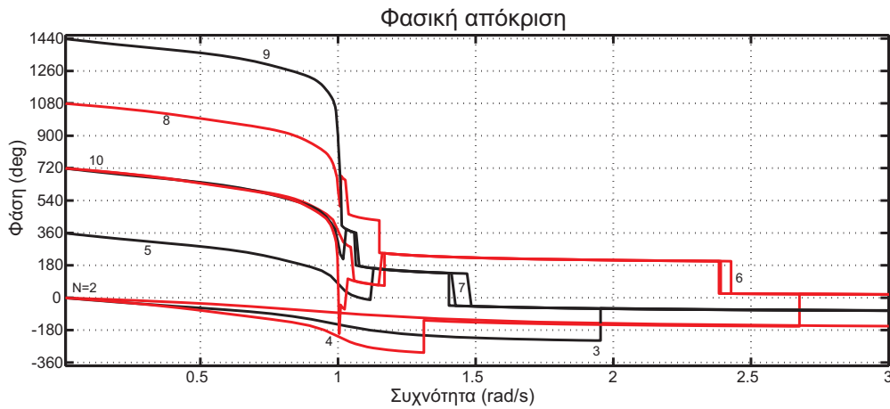
Σχήμα 0-7 Η φασική απόκριση του πρωτότυπου χαμηλοπερατού ελλειπτικού φίλτρου για συχνότητα αποκοπής \omega_c = 1 , τιμές παραμέτρων A_p = 1 dB, A_s = 30 dB και τιμές τάξης N = 1 έως N = 10 .
