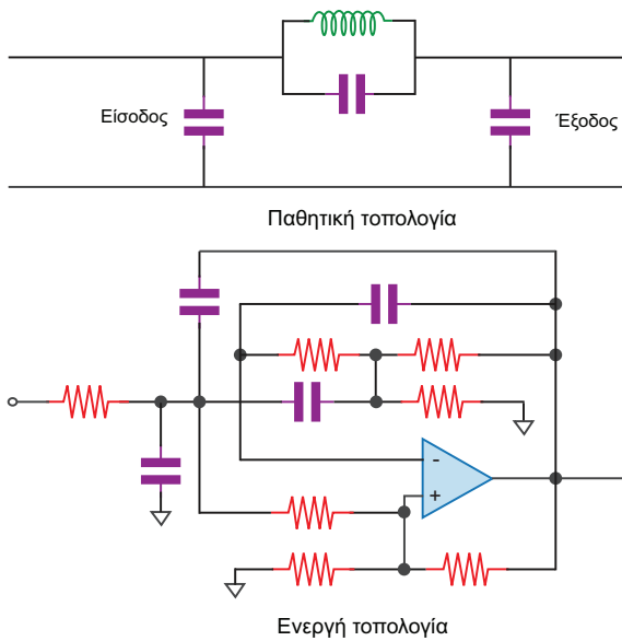
Σχήμα 0-2 Παράδειγμα παθητικού και ενεργού ελλειπτικού φίλτρου τρίτης τάξεως.
