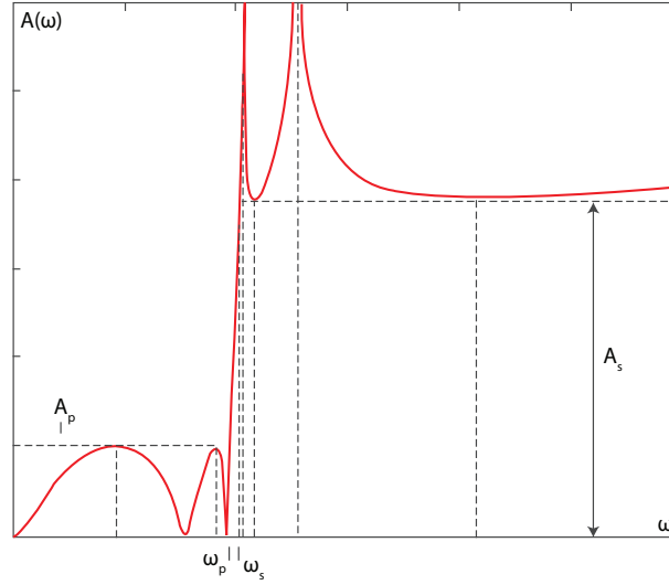
Σχήμα 0-6 Χαρακτηριστική απωλειών για ένα ελλειπτικό χαμηλοπερατό φίλτρο πέμπτης τάξεως.
