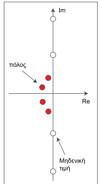
Σχήμα 0-5 Διάγραμμα πόλων μηδενικών τιμών χαμηλοπερατού ελλειπτικού φίλτρου τετάρτης τάξεως.
