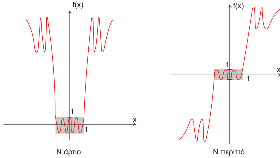
Σχήμα 0-4 Η ρητή συνάρτηση Chebyshev.
