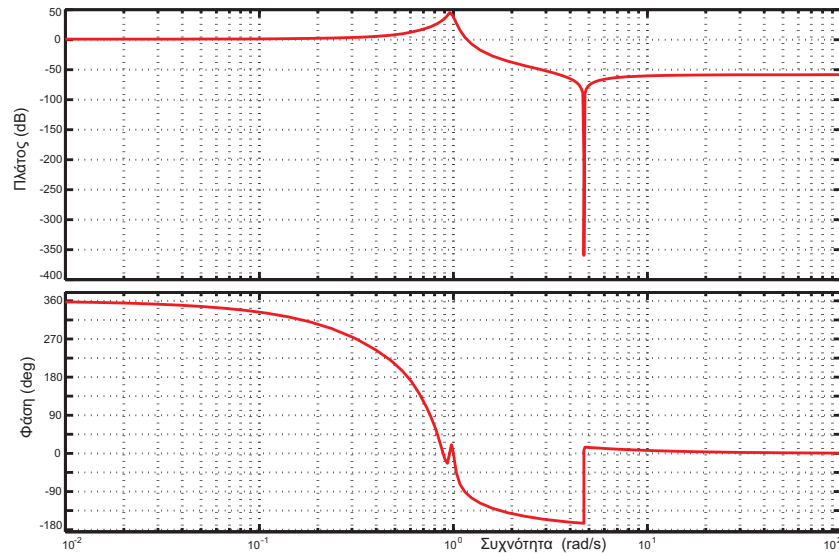
Σχήμα 0-9 Οι αποκρίσεις πλάτους και φάσης του ελλειπτικού φίλτρου της Άσκησης ??.
