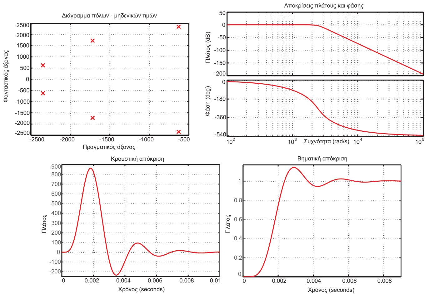
Σχήμα Α. Το διάγραμμα πόλων - μηδενικών τιμών, οι αποκρίσεις πλάτους και φάσης και η κρουστική και η βηματική απόκριση του χαμηλοπερατού φίλτρου της άσκησης.
