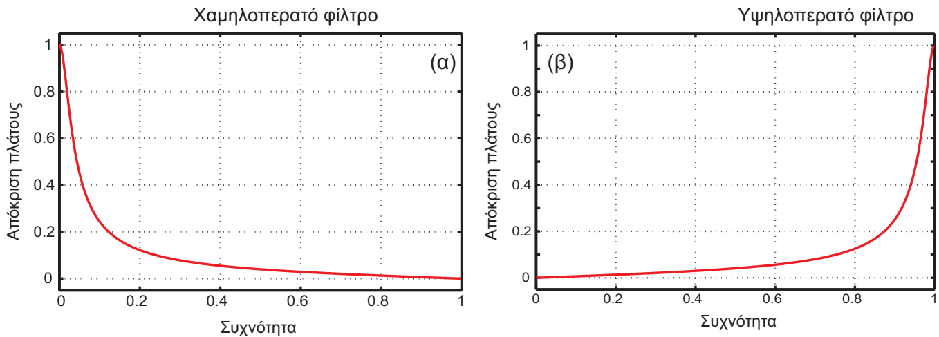
Σχήμα Α. Η απόκριση πλάτους του χαμηλοπερατού και υψηλοπερατού φίλτρου του Παραδείγματος 3.
