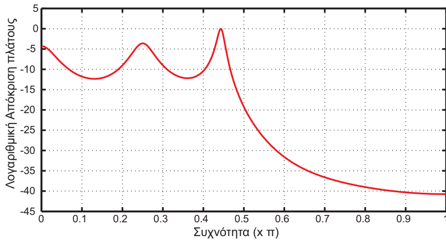
Σχήμα Α. Η απόκριση πλάτους του προσεγγιστικού χαμηλοπερατού φίλτρου που κατασκευάστηκε διά της εφαρμογής της μεθόδου του Padé για τιμές παραμέτρων M = 5 και N = 5 .
