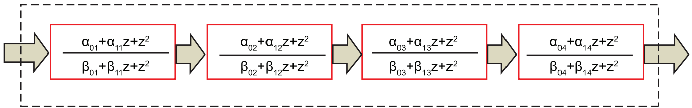
Σχήμα 0-3 Η σύνθεση του ψηφιακού αναδρομικού φίλτρου τάξεως N = 8 από τη εν σειρά σύνδεση τεσσάρων φίλτρων δευτέρας τάξεως.
