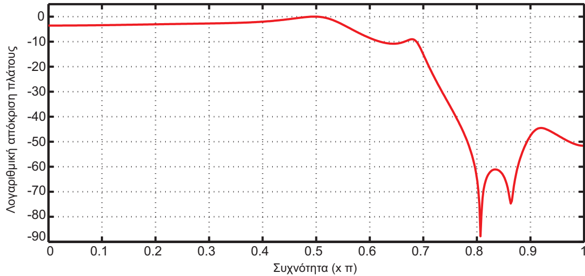
Σχήμα 0-4 Η απόκριση πλάτους του ψηφιακού αναδρομικού φίλτρου του Παραδείγματος 16.
