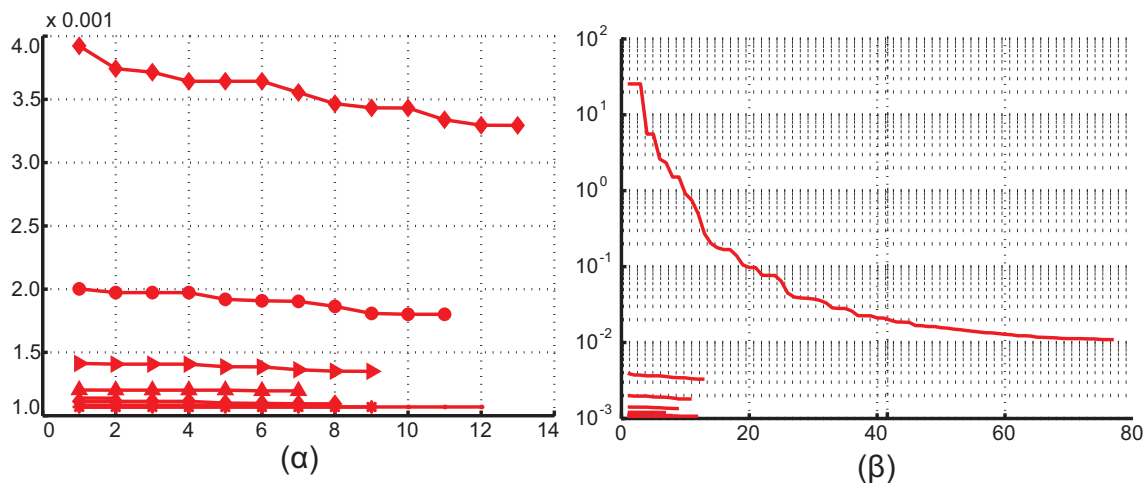
Σχήμα 0-2 Προσέγγιση του ελαχίστου της αντικειμενικής συνάρτησης από τη συνάρτηση f_{\min} συναρτήσει του αριθμού επανάληψης k του αλγορίθμου βελτιστοποίησης.
