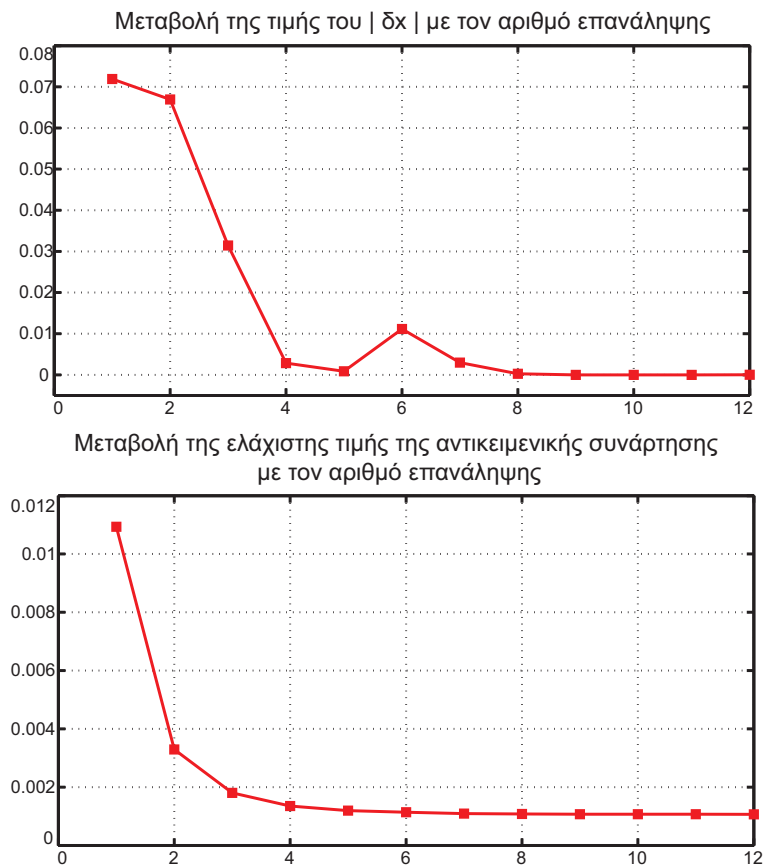
Σχήμα 0-1 Η μεταβολή του μέτρου της διαφοράς |\delta x| των διαδοχικών διανυσμάτων και της ελάχιστης τιμής της αντικειμενικής συνάρτησης \Psi(x_k)_{\min} συναρτήσει του αριθμού επανάληψης k .
