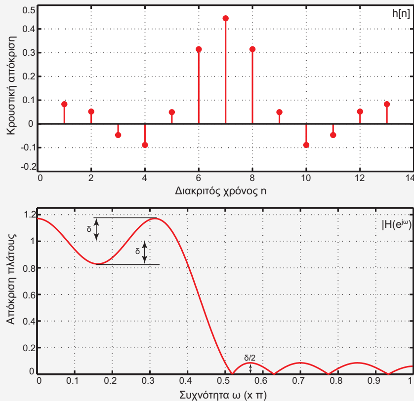
Σχήμα 0-3 Η κρουστική απόκριση και η απόκριση πλάτους του φίλτρου της Άσκησης ??.
