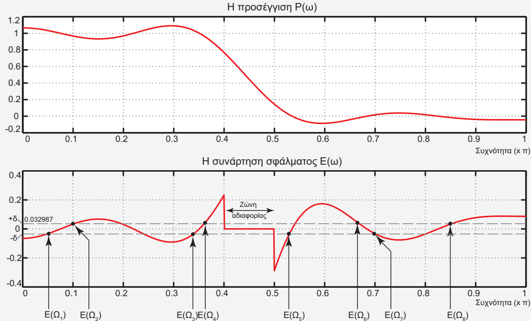
Σχήμα 0-1 Η προσέγγιση \mathcal{P}(\omega) και η συνάρτηση σφάλματος \mathcal{E}(\omega) μετά το τέλος της πρώτης επανάληψης. Από το σχήμα παρατηρούμε πως η συνάρτηση σφάλματος στη θέση του τρέχοντος συνόλου αναφοράς λαμβάνει την ίδια τιμή αλλά με εναλλασσόμενο πρόσημο, σε πλήρη συμφωνία με το θεώρημα της εναλλαγής.
