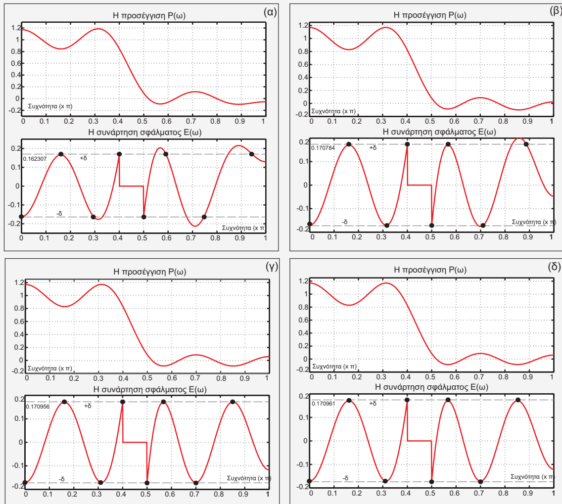
Σχήμα 0-2 Η καμπύλη των συναρτήσεων \mathcal{P}(\omega) και \mathcal{E}(\omega) για τις επαναλήψεις 2 [εικόνα (α)], 3 [εικόνα (β)], 4 [εικόνα (γ)] και 5 [εικόνα (δ)].
