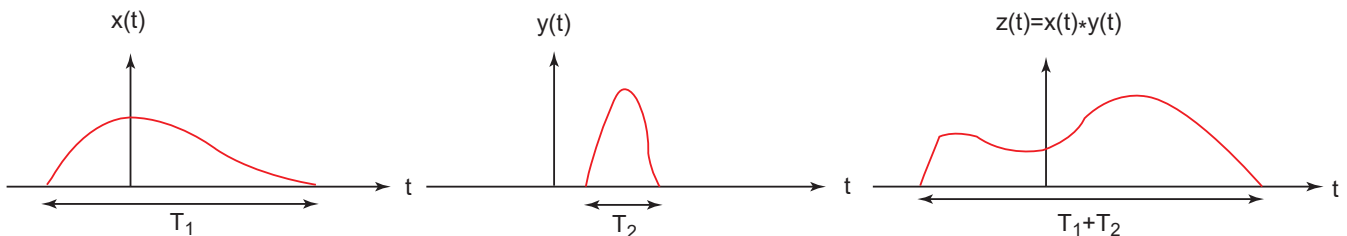
Σχήμα Α. Γραφική επίδειξη της ιδιότητας του εύρους της συνέλιξης σημάτων πεπερασμένης διάρκειας.
