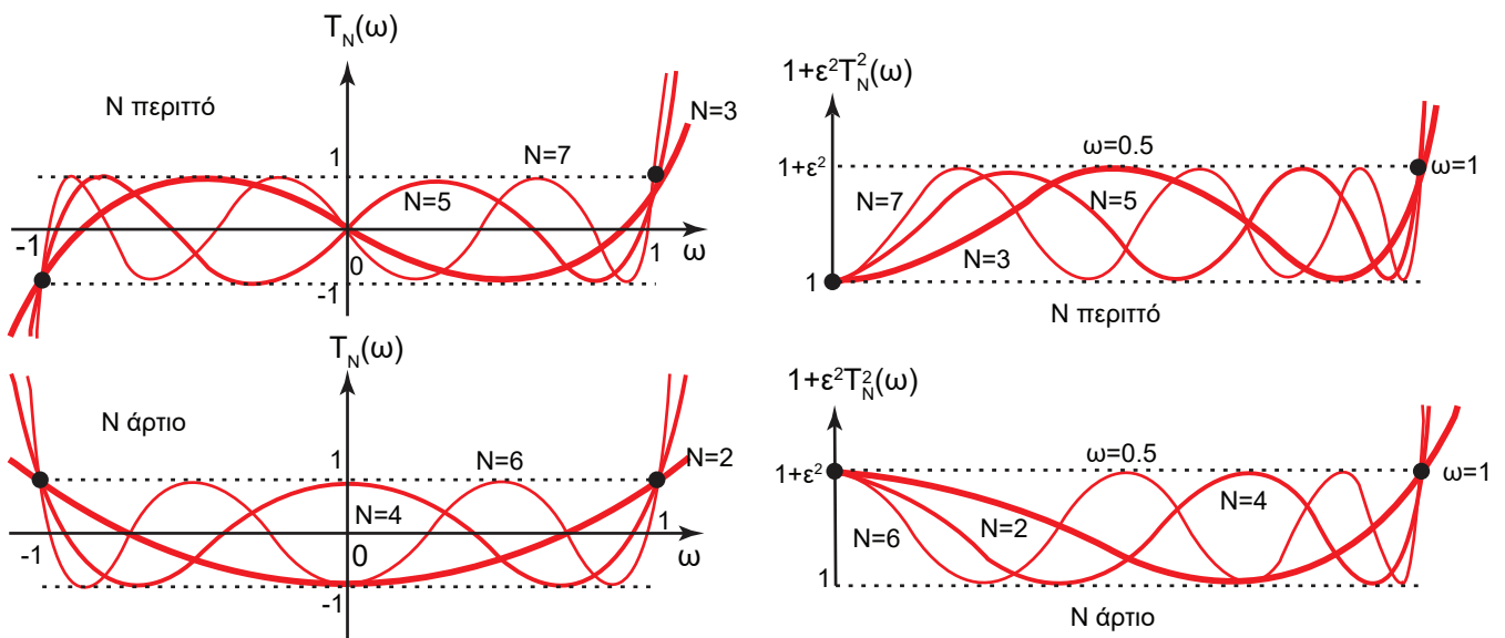
Σχήμα 1 Τα πολυώνυμα Chebyshev πρώτου είδους βαθμού N για διάφορες άρτιες και περιττές τιμές τάξης και η αντίστοιχη συνάρτηση 1 + T_N^2(\omega) .
