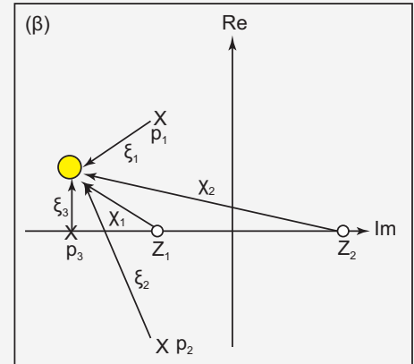
Σχήμα Α. Γεωμετρικός υπολογισμός της συνάρτησης \mathcal{H}(s) στις θέσεις s_1 = 3 + 5j και s_2 = -4 + j .
