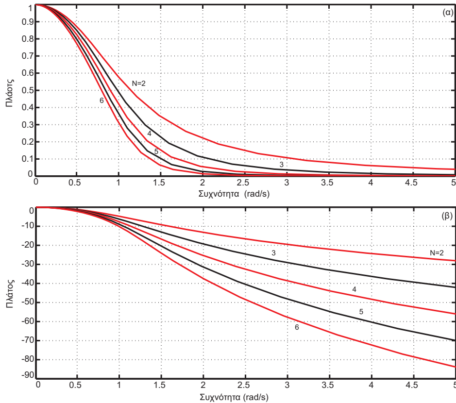
Σχήμα 2 Η απόκριση πλάτους του πρωτότυπου φίλτρου Bessel για τιμές τάξης φίλτρου N = 2, 3, 4, 5, 6 σχεδιασμένη στη γραμμική κλίμακα [εικόνα (α)] και στη λογαριθμική κλίμακα [εικόνα (β)]. Σε αμφότερα τα διαγράμματα ο οριζόντιος άξονας των συχνοτήτων είναι βαθμονομημένος στη γραμμική κλίμακα.
