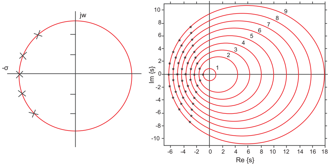
Σχήμα 5 Πόλοι φίλτρου Bessel για την κανονικοποιημένη και μη κανονικοποιημένη περίπτωση. Στην αριστερή εικόνα η τάξη του φίλτρου είναι N = 5 , ενώ στη δεξιά εικόνα κυμαίνεται από N = 1 έως N = 10 . Σε πλήρη αναλογία με τις προηγούμενες προσεγγίσεις ιδανικών φίλτρων, τα φίλτρα άρτιας τάξης διαθέτουν N/2 ζεύγη συζυγών μιγαδικών πόλων, ενώ τα φίλτρα περιττής τάξης ένα πραγματικό αρνητικό πόλο και (N - 1)/2 ζεύγη συζυγών μιγαδικών πόλων.
