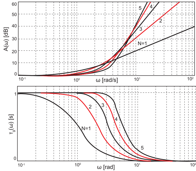
Σχήμα 1 Η μεταβολή της εξασθένισης και της υστέρησης ομάδας σε συνάρτηση με το μέγεθος της συχνότητας για ένα φίλτρο τύπου Bessel-Thomson.
