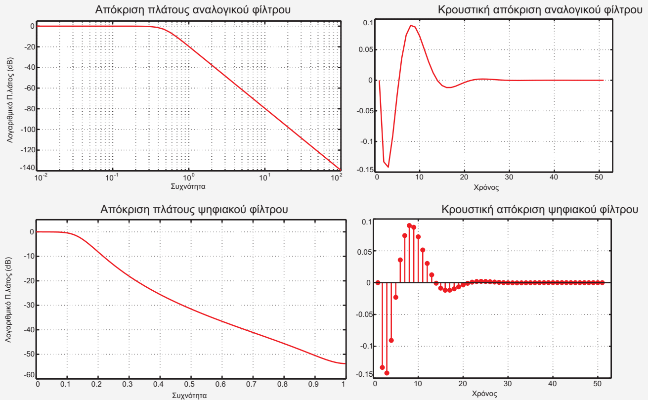
Σχήμα Α. Η συχνотική και η κρουστική απόκριση του αναλογικού φίλτρου και του αντίστοιχου ψηφιακού φίλτρου.
