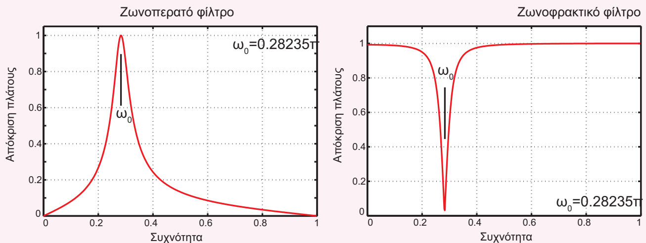
Σχήμα Α. Η απόκριση πλάτους του ζωνοπερατού και του ζωνοφρακτικού φίλτρου του παραδείγματος.
