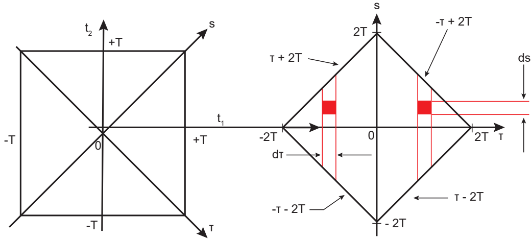
Σχήμα 2 Η γεωμετρία του προβλήματος κατανόησης της φασματικής πυκνότητας ισχύος (Stark & Woods, Σχήμα 7.5-1).
