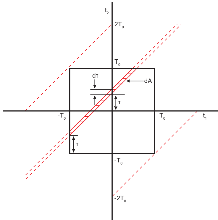
Σχήμα 1 Η γεωμετρία του προβλήματος υπολογισμού της φασματικής πυκνότητας ισχύος (Αντωνίου, Σχήμα 13.4).
