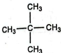
neo-Pentane
