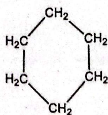
Cyclo hexane
