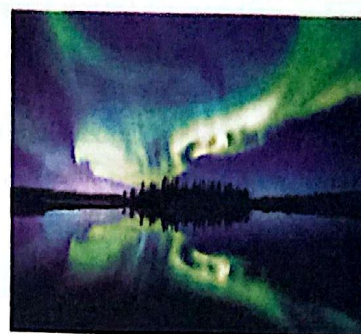
Aurora
