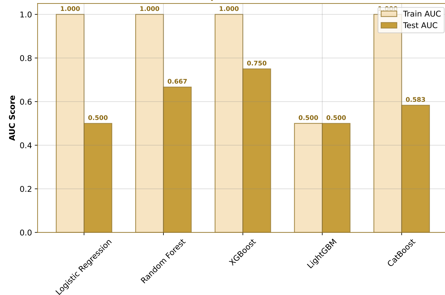
AUC Comparison: Train vs Test
