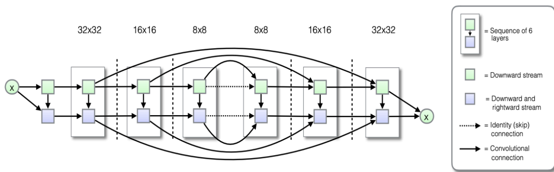
شکل ۲-۳: معماری pixelCNN++
