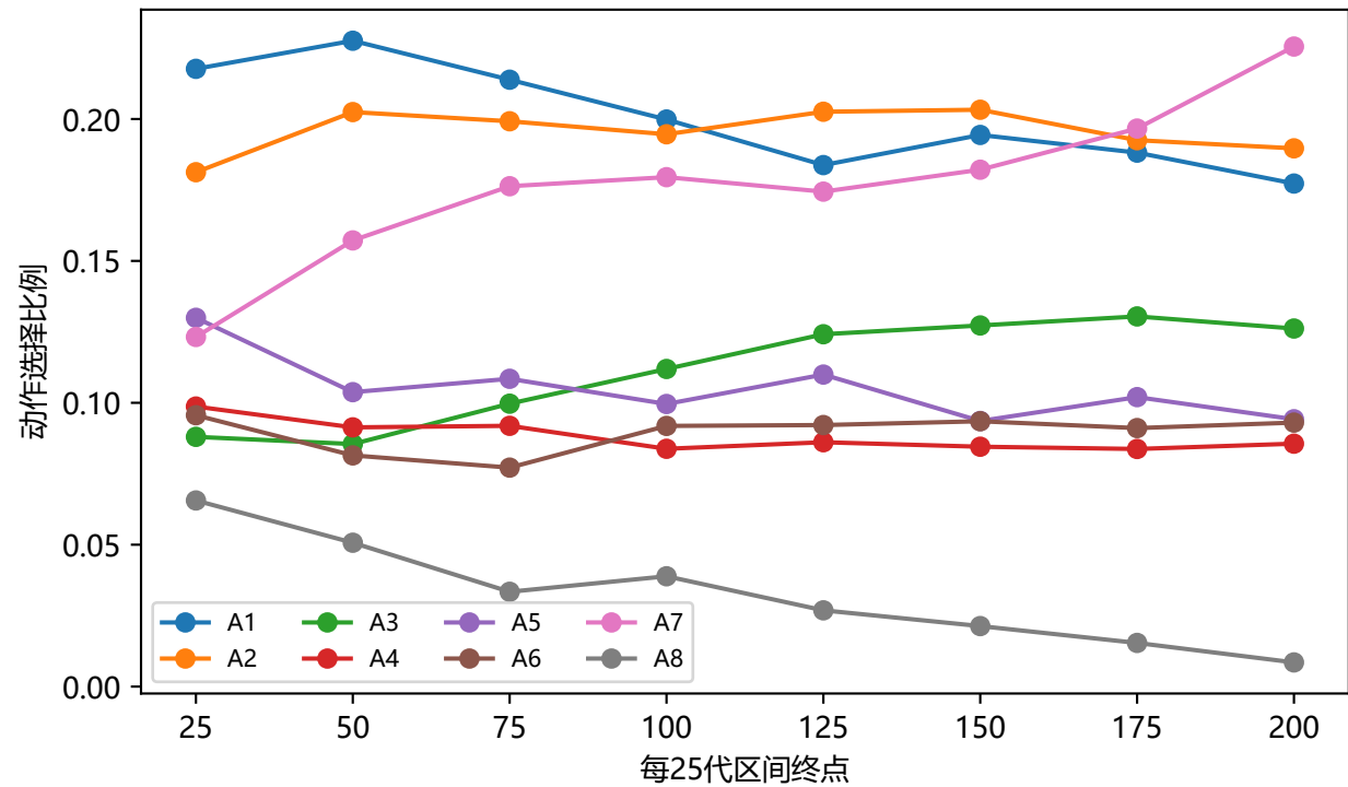
算子使用随搜索进程变化
