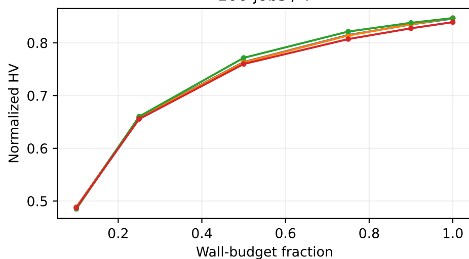
100 jobs / T
