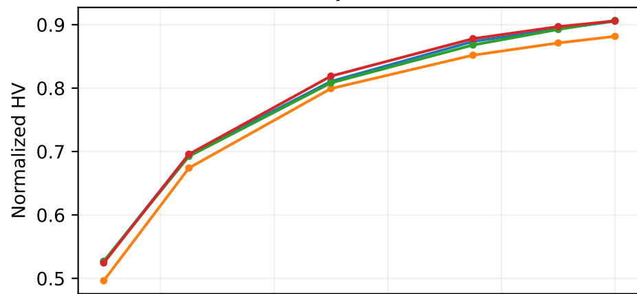
50 jobs / T
