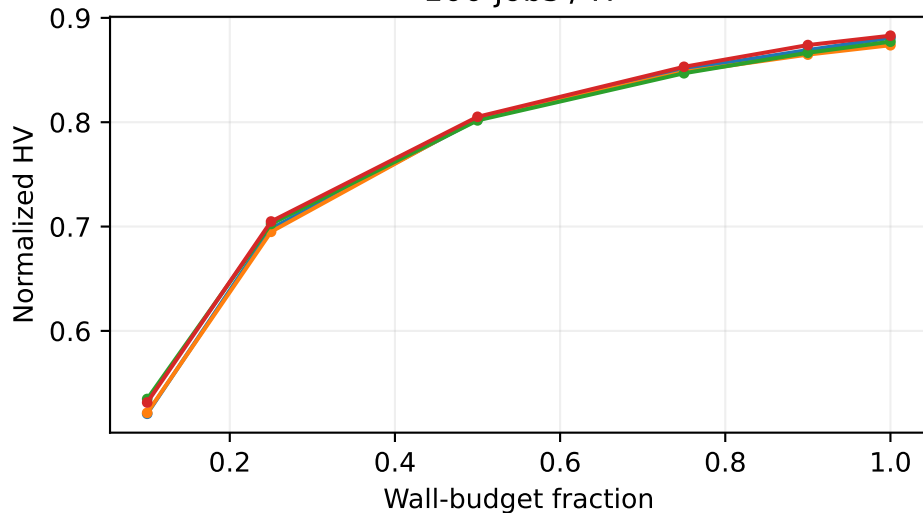
100 jobs / H
