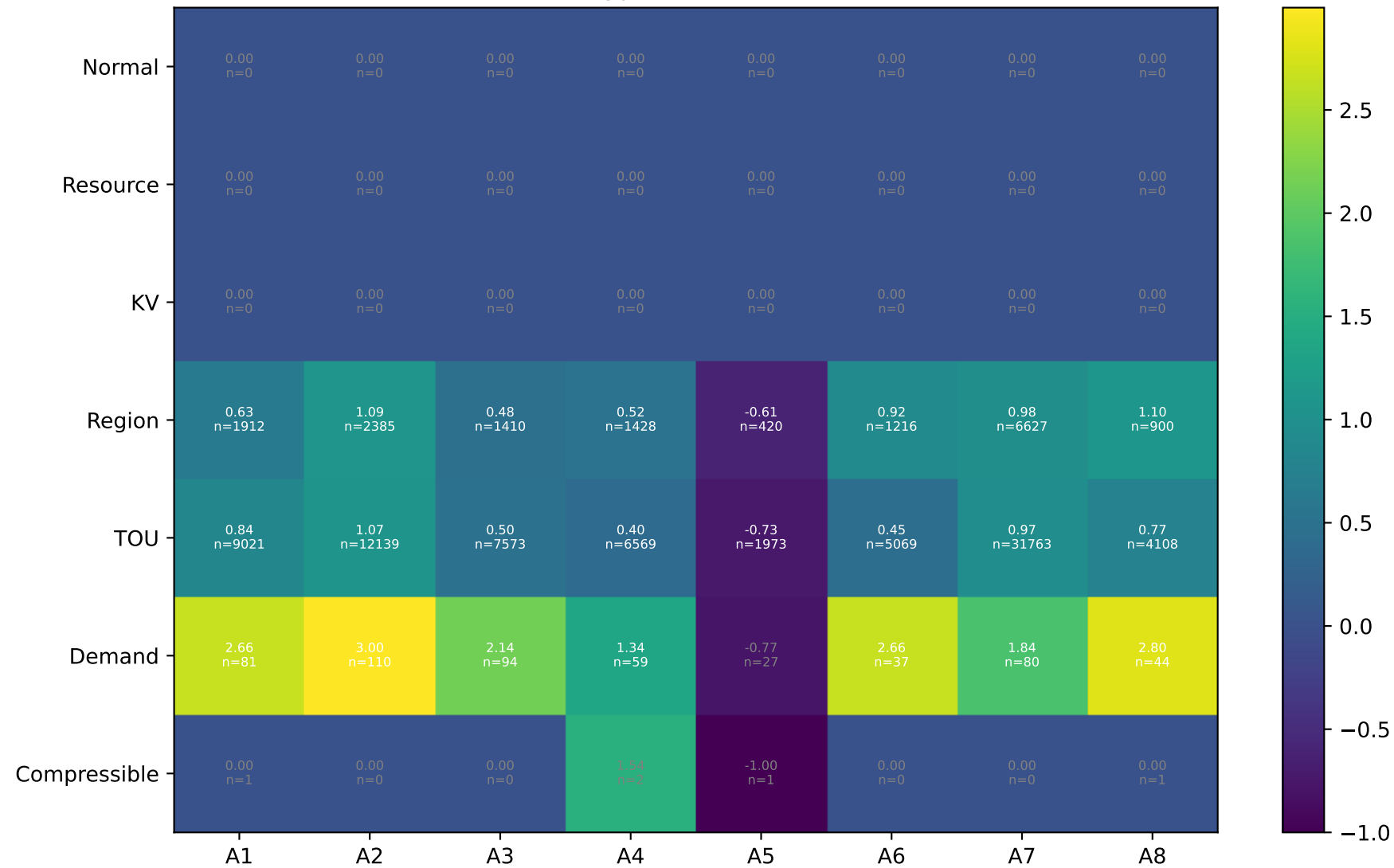
D03 Type-II: Mean reward
