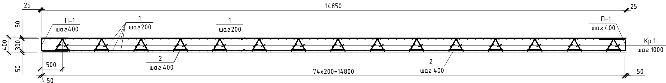
1-1 (армирование)
