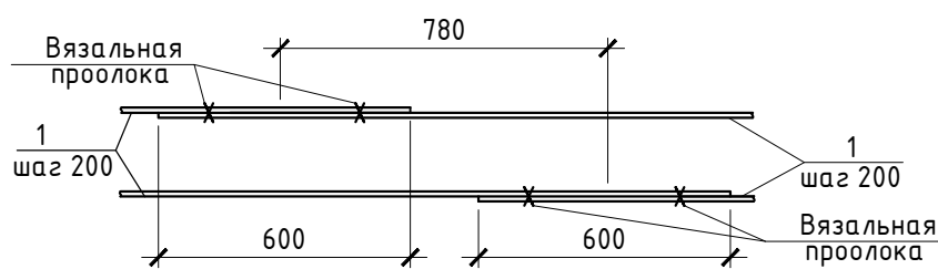
Узел стыка арматуры
