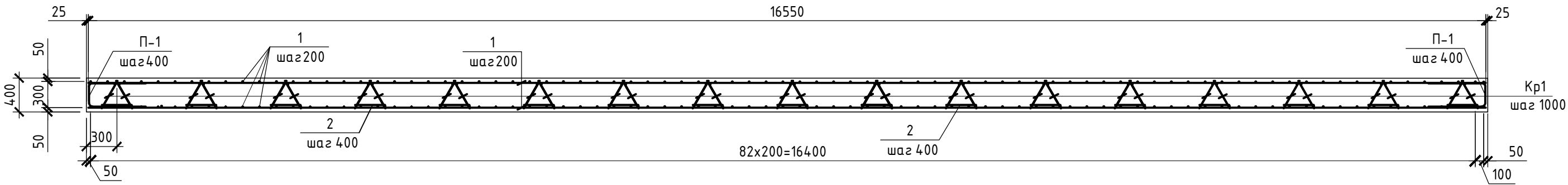
1-1(армирование)
