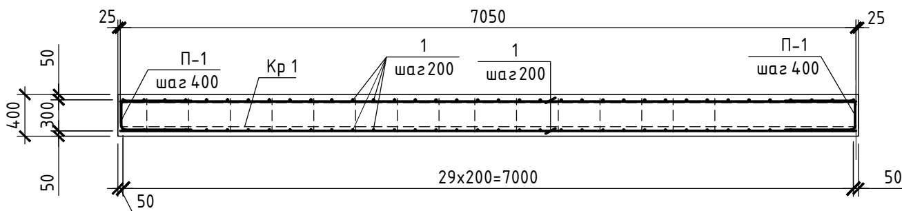
2-2 (армирование)
