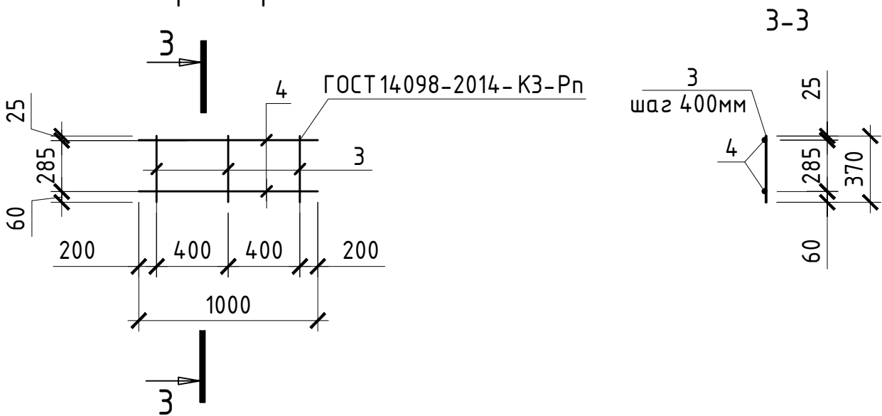
Каркас Кр1
