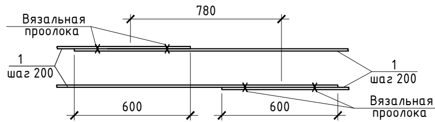
Узел стыка арматуры
