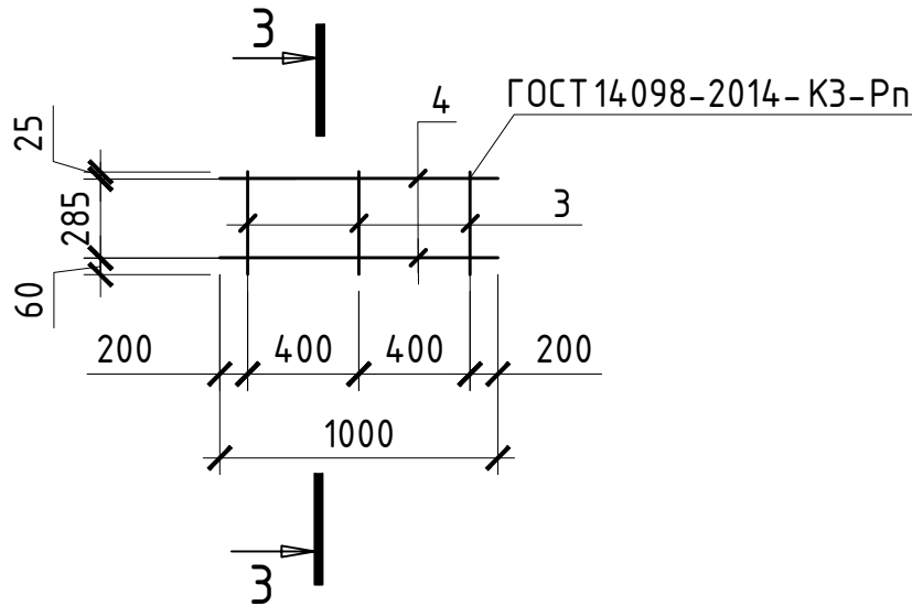
Каркас Кр1
