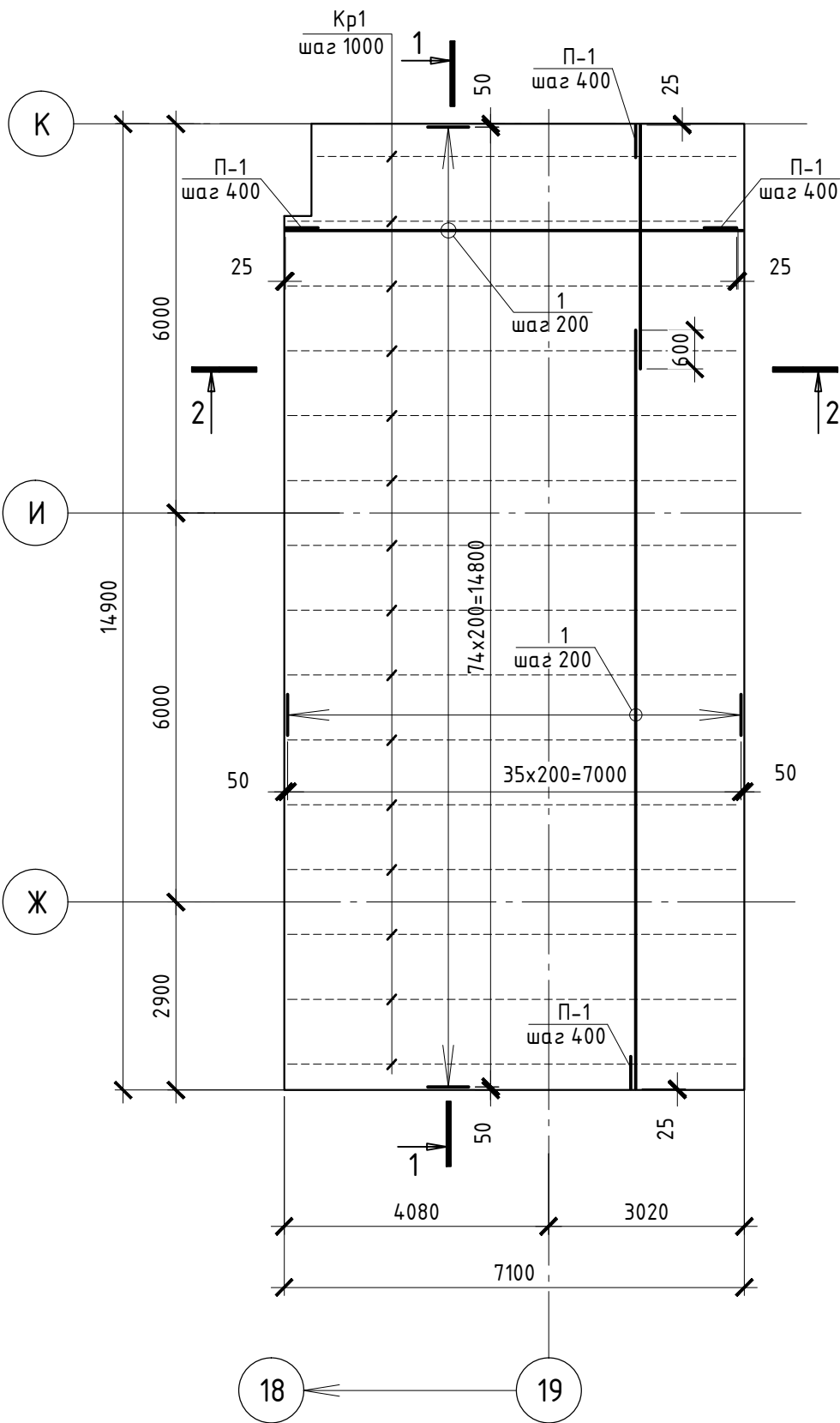
Фундамент ФМПЗ (армирование)
