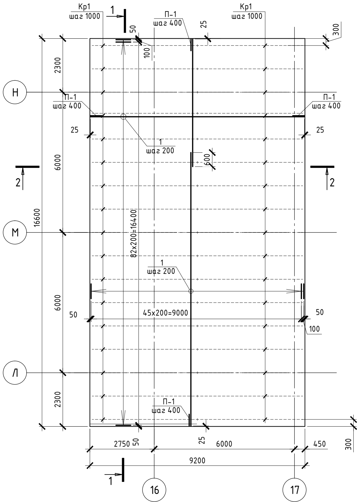
Фундамент ФМП2 (армирование)
