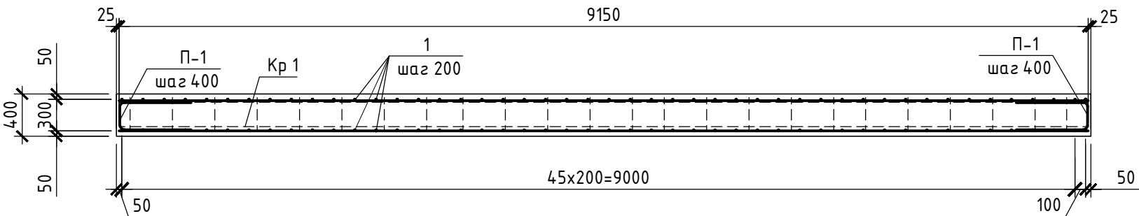
2-2(армирование)
