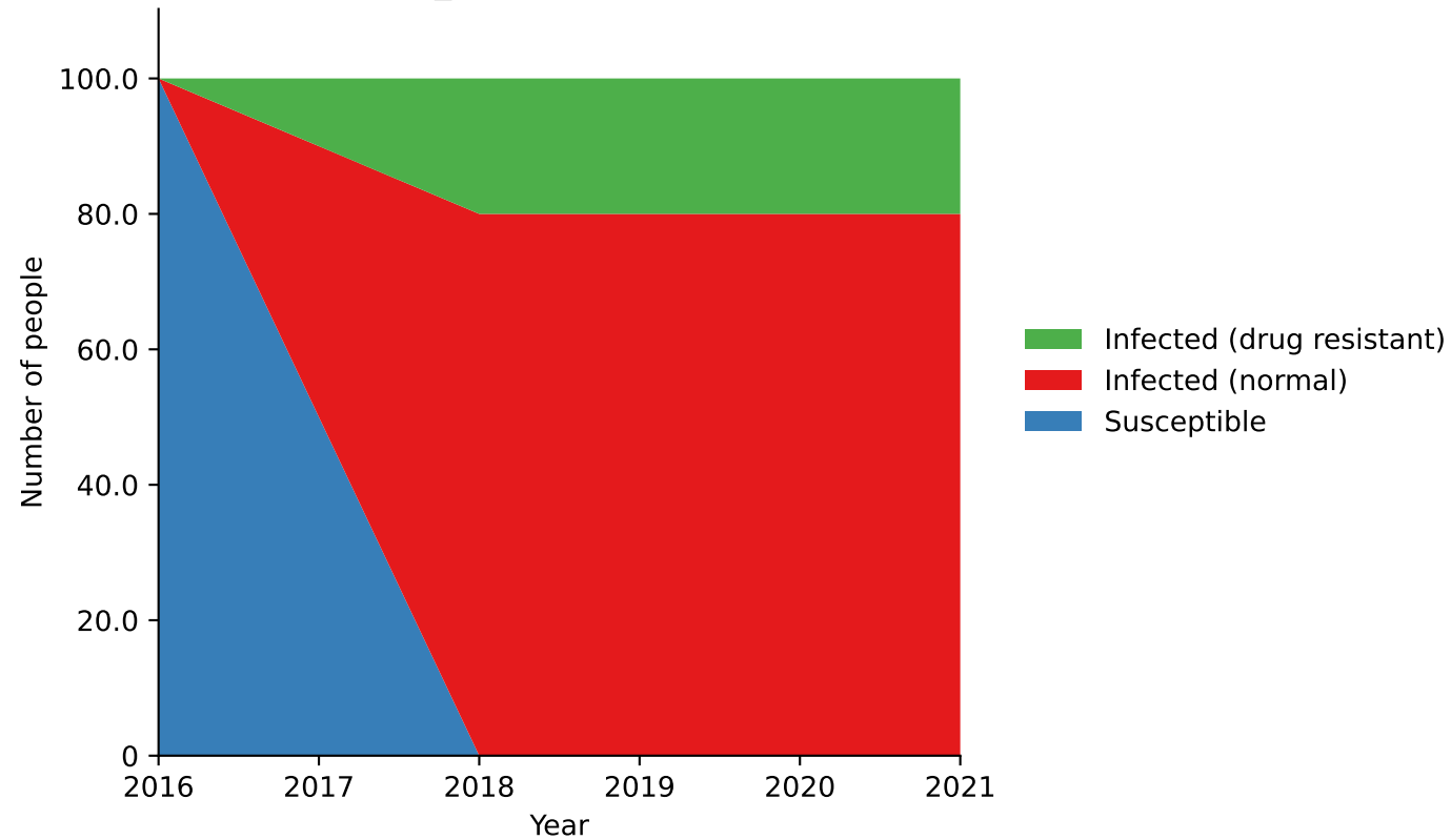
parset_default-Population 0
