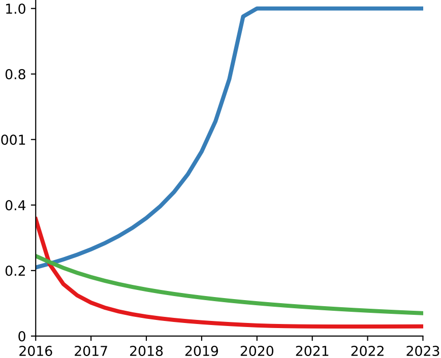
parset_default_1-m_rural
