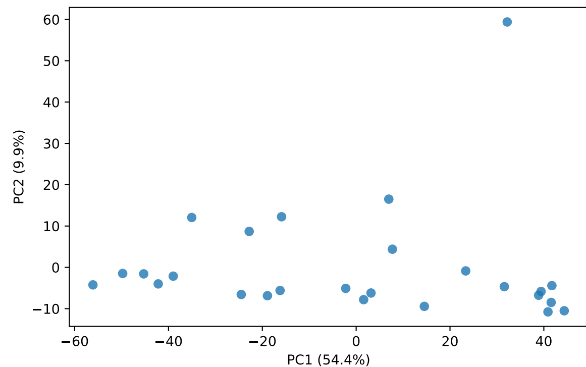
PCA Scores
