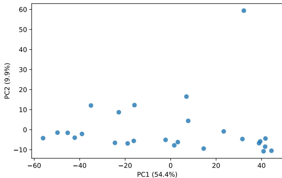
PCA Scores
