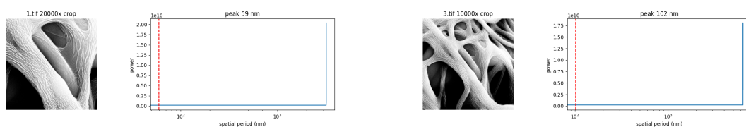
图 4.3: 表面条纹间距的 FFT 径向功率谱（左 20k，右 10k），虚线标出主峰周期（45–59 nm 与 \approx 102\text{ nm} ）。
