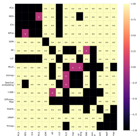
AMI
