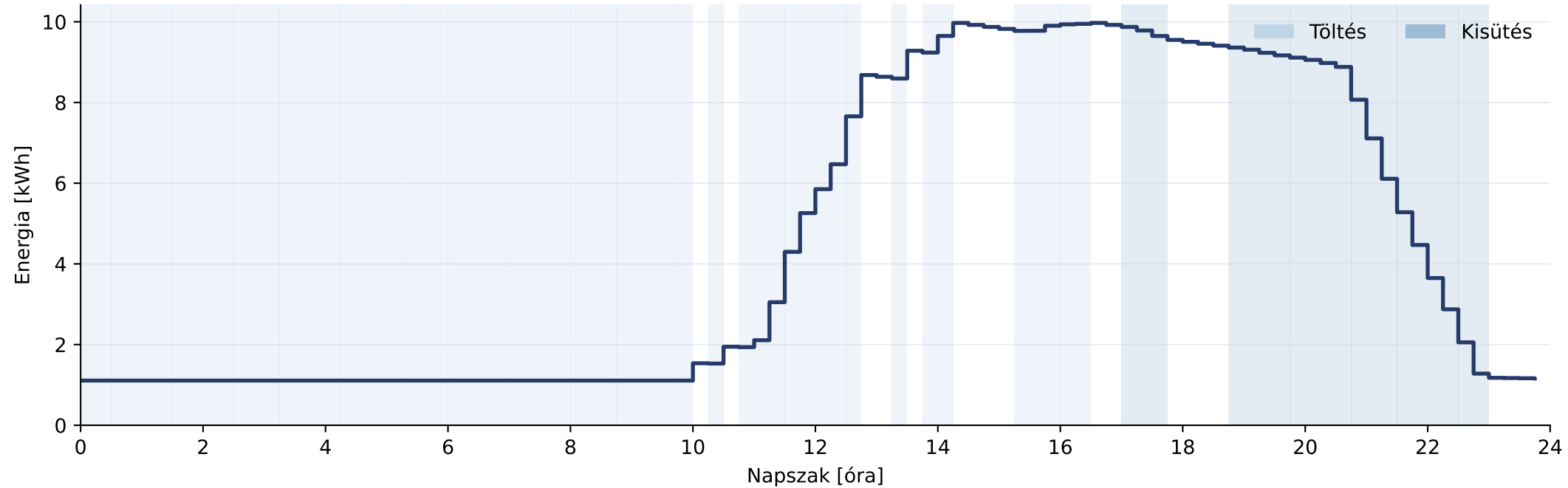
0420144888460007 | 2021-10-01 | Akkumulátor energiaszintje
