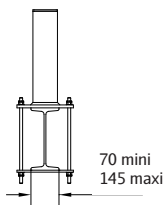
Fixation par bridage standard possible. Jeux grandes brides 305 mm maxi
