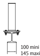
Fixation par crapautage
