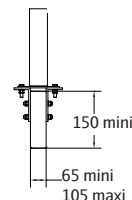
Fixation par cornières sur poutre lamellée collée
