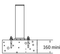
Fixation par scellements
