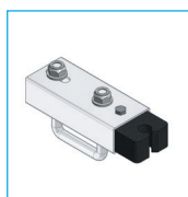
Guide-câble fixé par bridage sur les échelons grâce à un étrier
