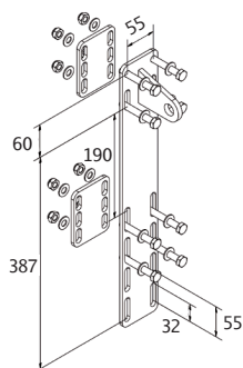
Platine supérieure
