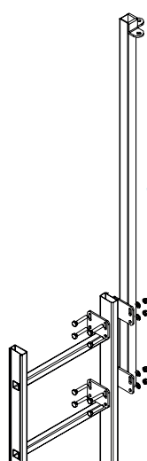
Extension fixation sur montant latéral
