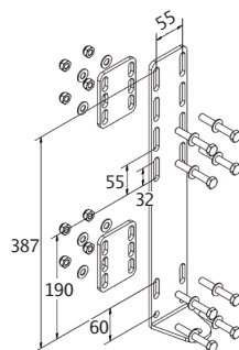
Platine inférieure
