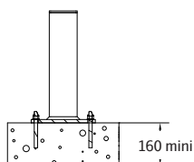
Fixation par scellements
