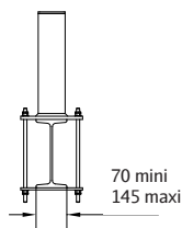
Fixation par bridage standard possible. Jeux grandes brides 305 mm maxi
