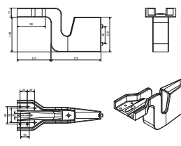
Platine Z moulée
