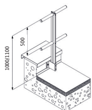
Eco-Line T22 en applique
