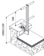
Eco-Line T22 sous couverture - acrotère non isolé
