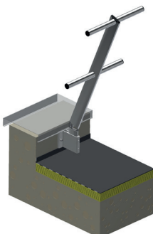
Support Eco-Line T22 incliné Fixation en applique (intérieur acrotère)
