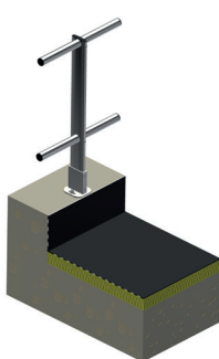
Support Eco-Line T22 Fixation sur dessus (acrotère non isolé)
