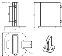
Platine sur dessus
