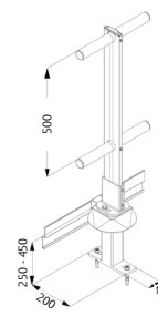
Eco-Line T22 sur potelet
