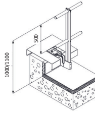
Eco-Line T22 sous couverture acrotère isolé
