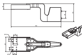
Platine Z rallongée
