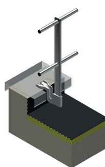
Support Eco-Line T22 Fixation sur platine Z sous couvertine (acrotère isolé ou non isolé)
