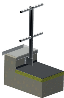
Support Eco-Line T22 Fixation en applique (intérieur acrotère)
