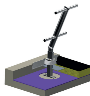
Support Eco-Line T22 incliné fixation sur potelet collerette plastique
