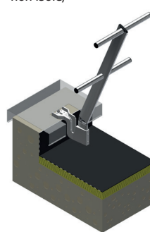
Support Eco-Line T22 incliné Fixation sur platine Z sous couvertine (acrotère isolé ou non isolé)
