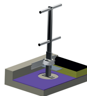
Support Eco-Line T22 sur potelet collerette plastique
