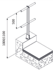
Eco-Line T22 sur dessus
