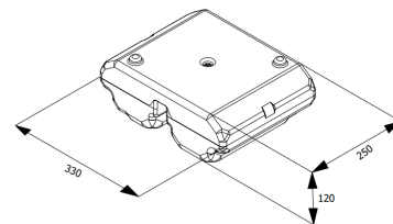
Plot béton avec poignée (12,5kg)
