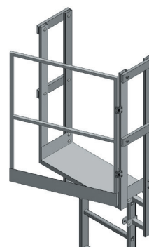
OPTION : marche palière et portillon
