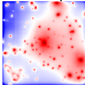
F850lp
