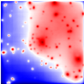
F606w
