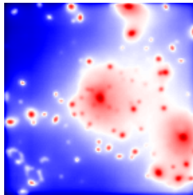
F814w
