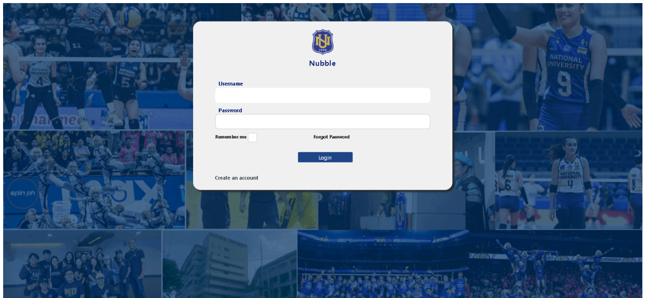
Figure 3.5.1: Login Module
