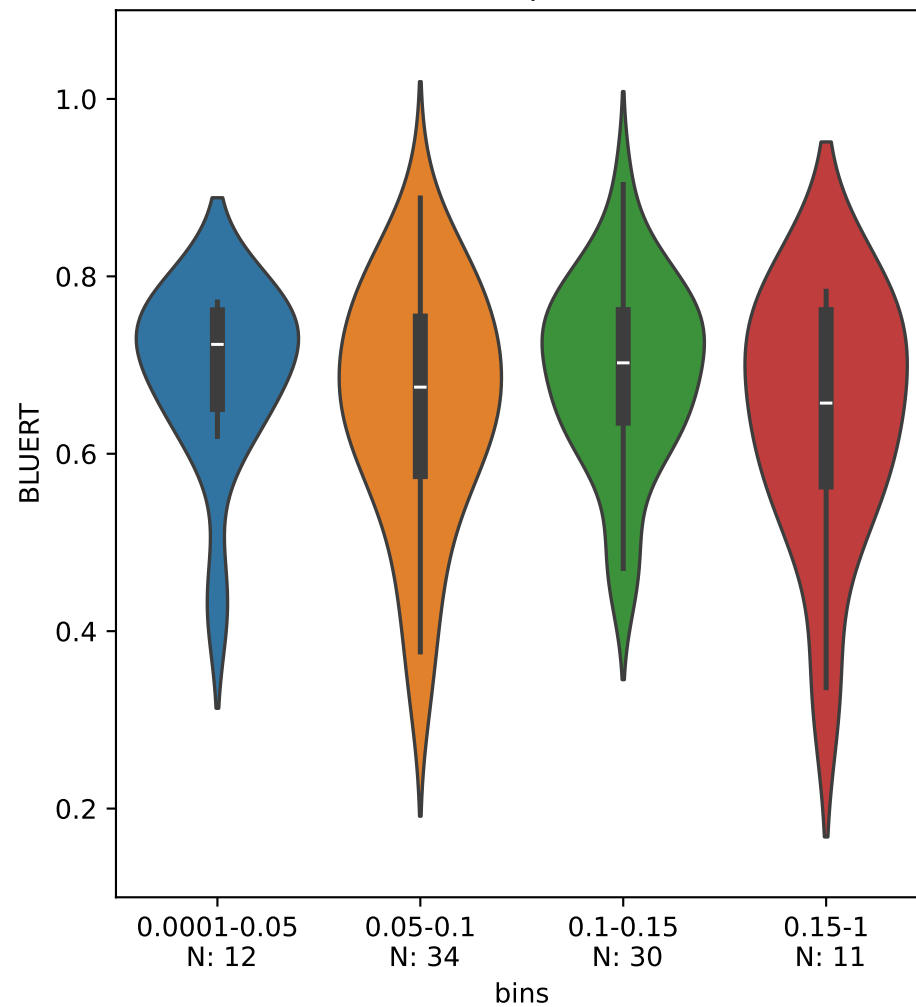
Token Swap BLEURT
