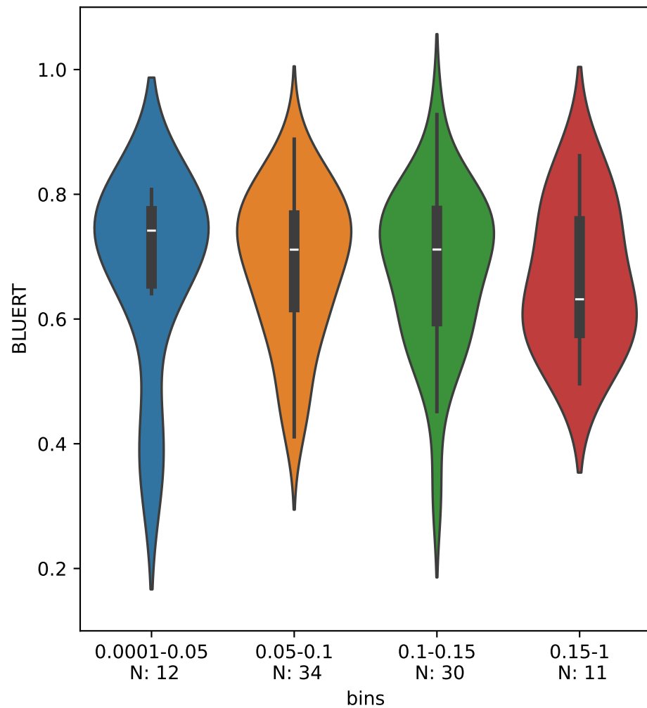
Baseline BLEURT
