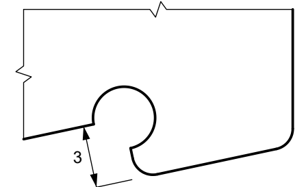
rebords du dessous, 2 ex. largeur (8,15) en projection ; degagement R1,5 comme B
