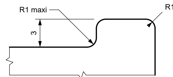
rebords du dessus, 2 ex. largeur (6,25) ; pied : angle de fraise, R1 maxi
